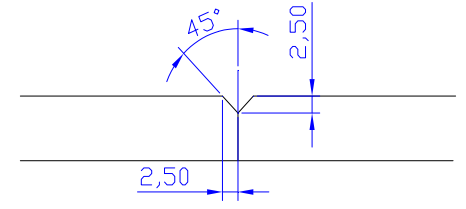
Schuine kant 45°
