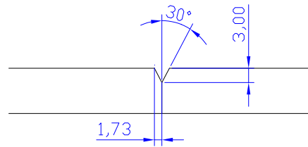
Schuine kant
